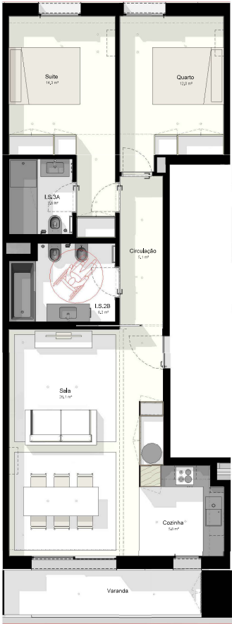
T2 - TIPO 1A 1 : 75
